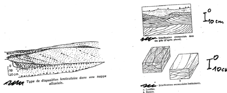
Fig 16 : Lentilles et litages entrecroisés
