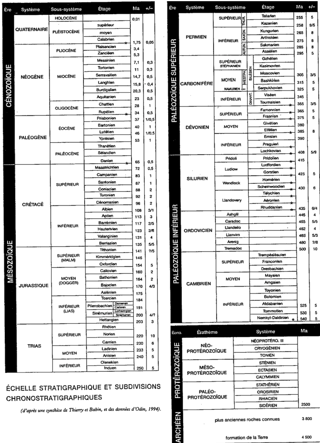
Fig. 26 Echelle internationale des temps géologiques
