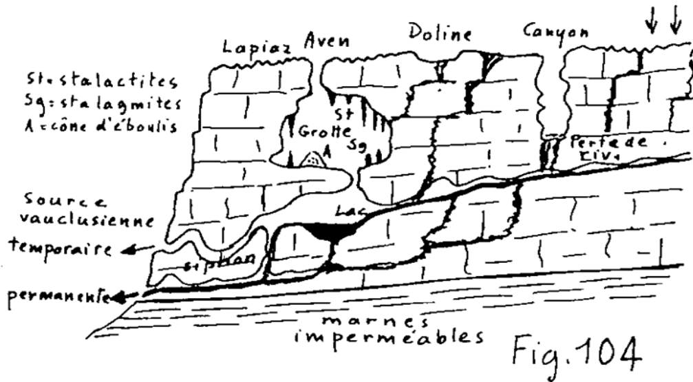
Fig. 28 : L'eau et les cavités dans les massifs de calcaires karstiques
