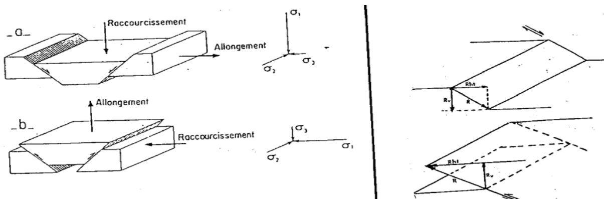
Fig. 25 Différents types de faille ; Rejet d'une faille - à gauche : les 3 principaux types de faille : a = normale ; b = inverse ; c = décrochement - à droite : le vecteur « rejet » ; en haut : faille normale ; en bas : faille inverse
