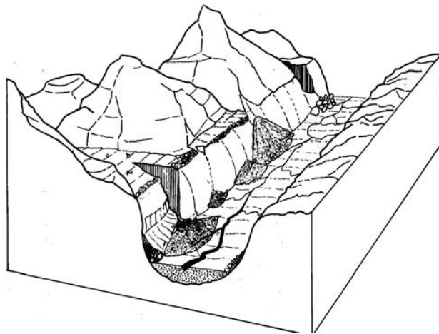
Fig. 13 Cônes d'éboulis et de déjections torrentielles dans une ancienne vallée glaciaire :
