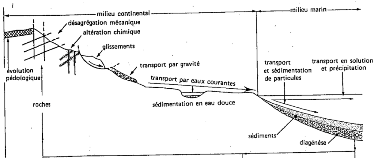
Fig. 12 Les processus sédimentaires
