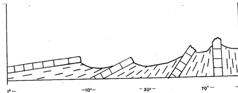
Fig. 23 Structures monoclinales :
