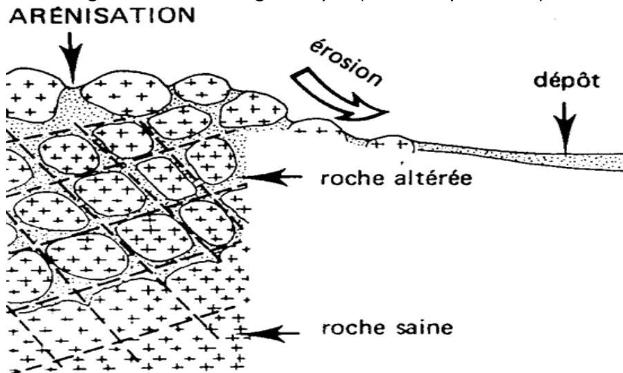
Fig 10 – Le phénomène d'arénisation d'un massif
