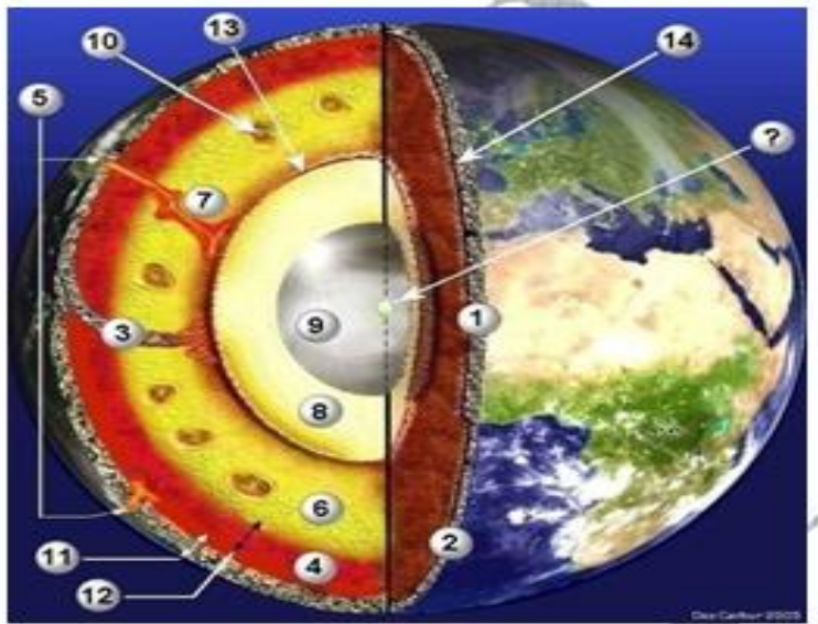
Figure 3 : Structure détaillée de la terre
