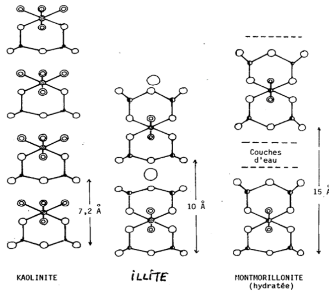
Figure n° 45 : Structure schématisée de quelques minéraux phylliteux
