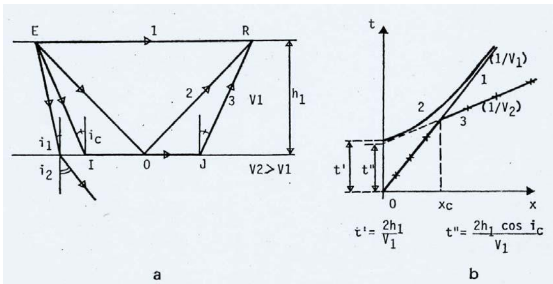
Fig. 27 : Propagation des ondes sismiques dans un milieu bicouche à interface parallèle à la surface
