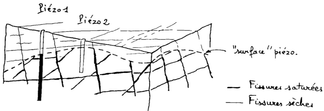
Fig. 29: La notion de nappe en milieu fissuré
