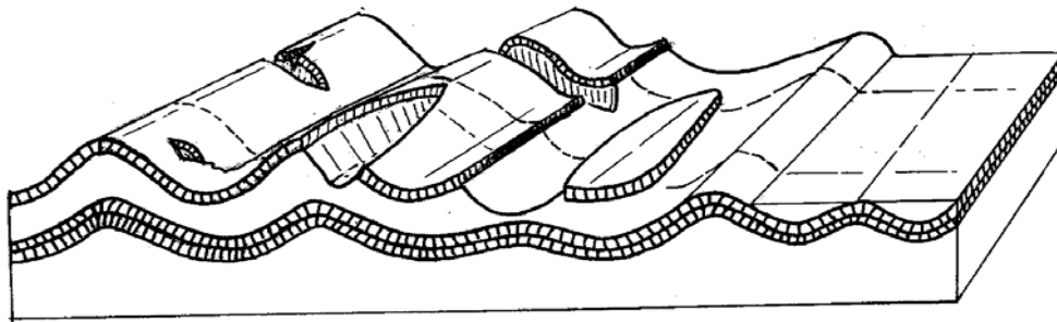
Fig. 24 Structures plissées : - à gauche : structure classique de relief jurassien, anticlinaux en relief attaqués par l'érosion - à droite : relief « inversé », classique en cas d'érosion importante
