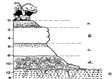
Fig.11 Coupe en terrain latéritique
