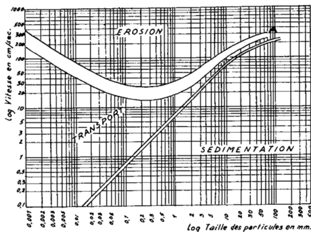
Fig. 14 : Diagramme de Hjulström : les processus sédimentaires (Erosion-Transport-Sédimentation) en fonction de la taille des particules et de la vitesse du courant (échelles log)
