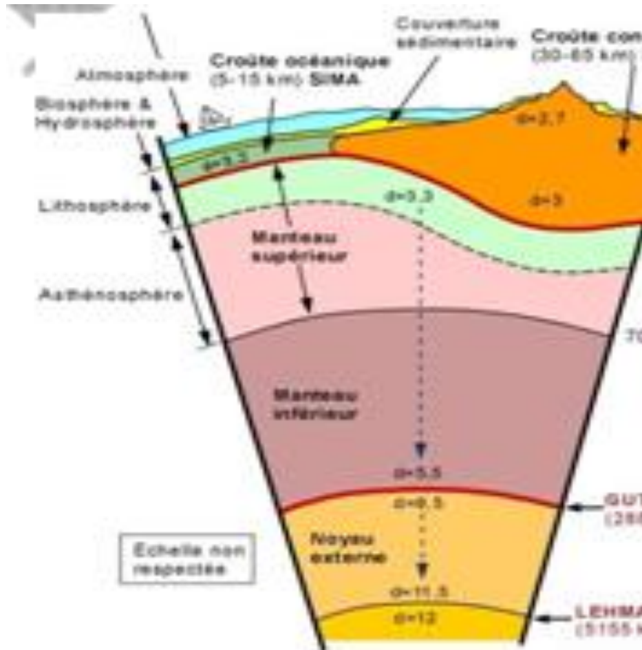
Figure 2 : Détail de la Lithosphère et de l'asthénosphère
