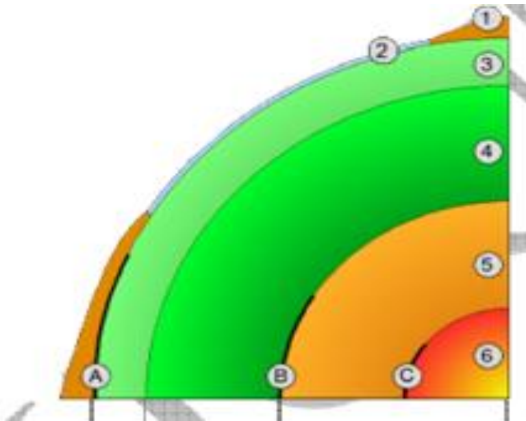
Figure 1 : Structure interne de la Terre
