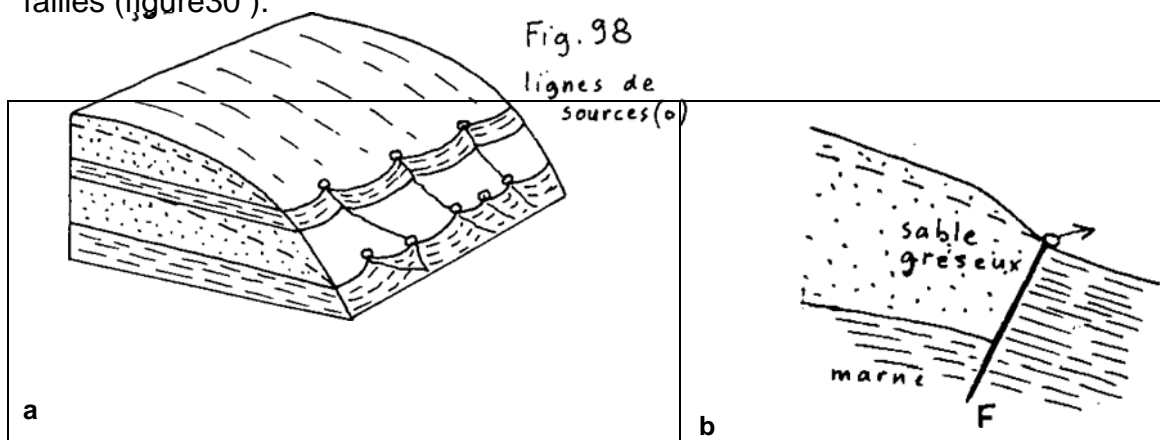
Fig. 30 : Exemples de sources a : contact stratigraphique ; b : faille
