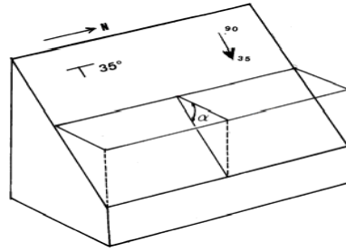
Fig. 21 Définition géométrique des plans géologiques éologiques
